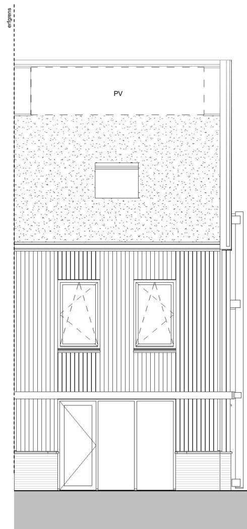
achtergevel
