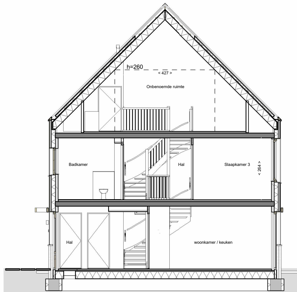
doorsnede
